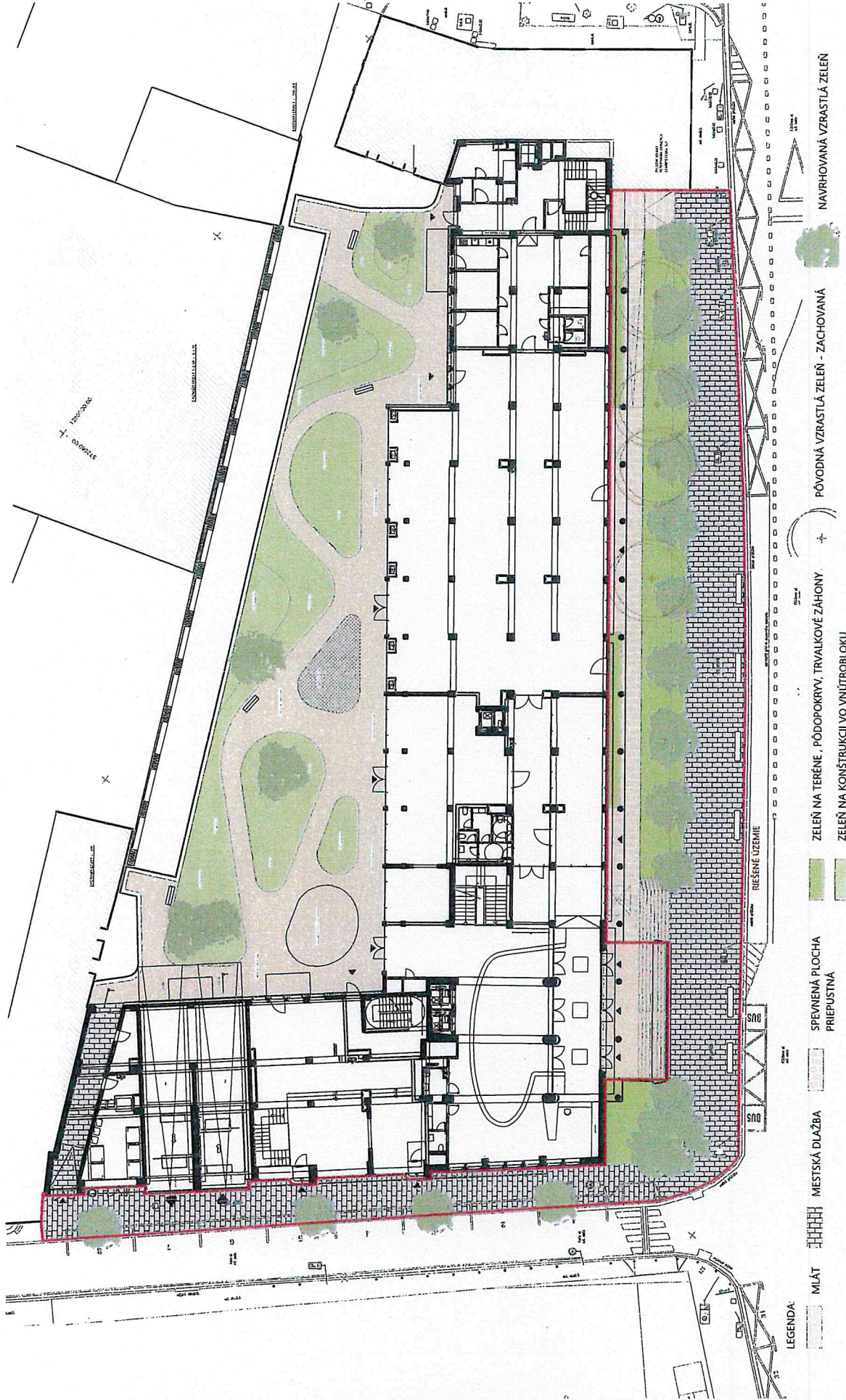
PÓDORYS - NÁVRH ÚPRAVY PREDPOLIA A OKOLITÝCH SPEVNENÝCH PLOCH V SÚVISLOSTI SO ZMENOU STAVBY STAROMESTSKÁ 6 M=1:250
