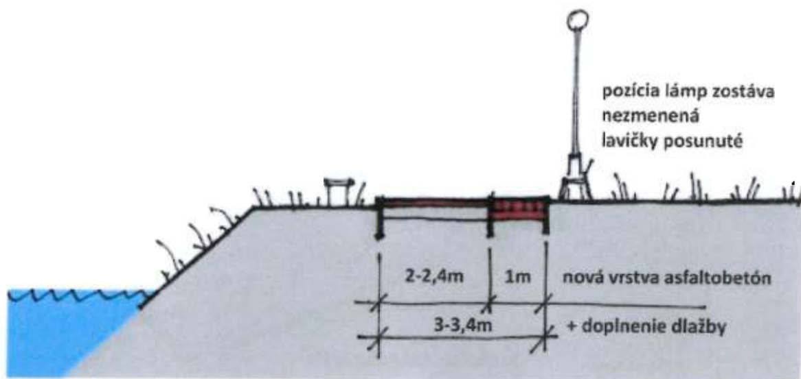
asfaltobetón
