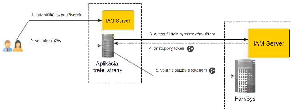
Obrázok 1: Autorizácia volaní ParkSys Web API systémovým účtom
